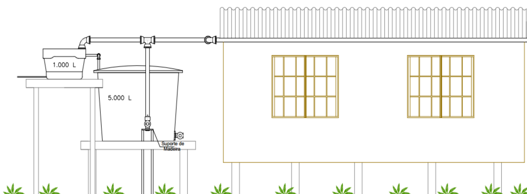
Figura 6: Desenho esquemático do componente complementar e componentes de captação de água de chuva.
