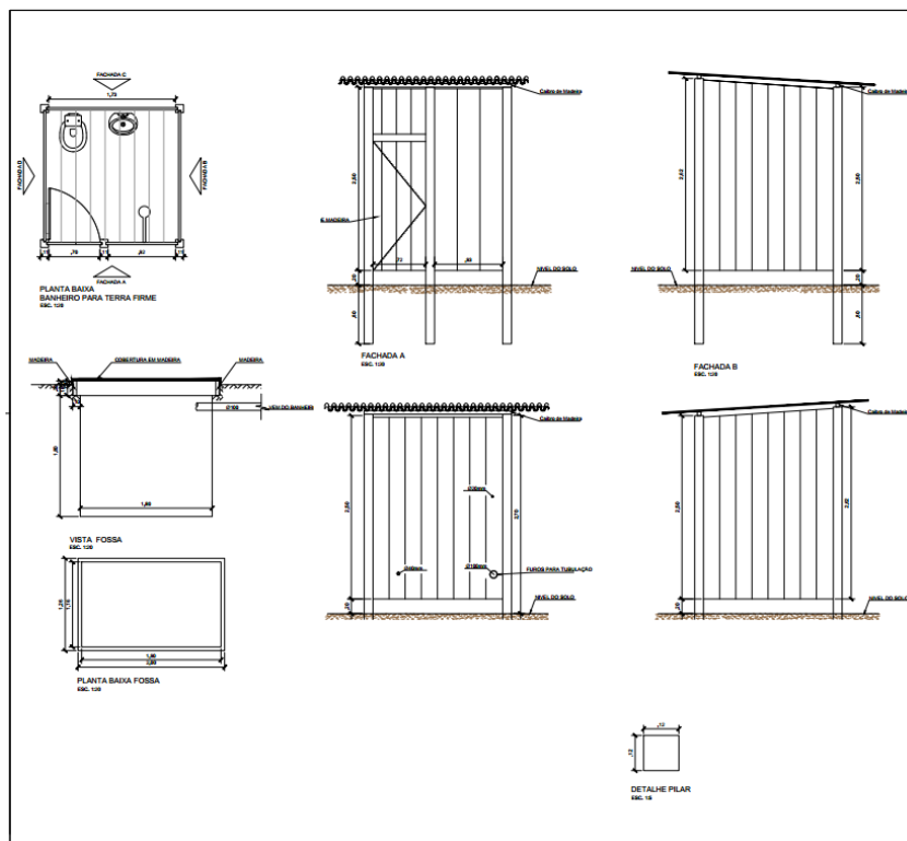
Figura 2: Instalação Sanitária Domiciliar de madeira adequada para ambiente de Terra Firme
