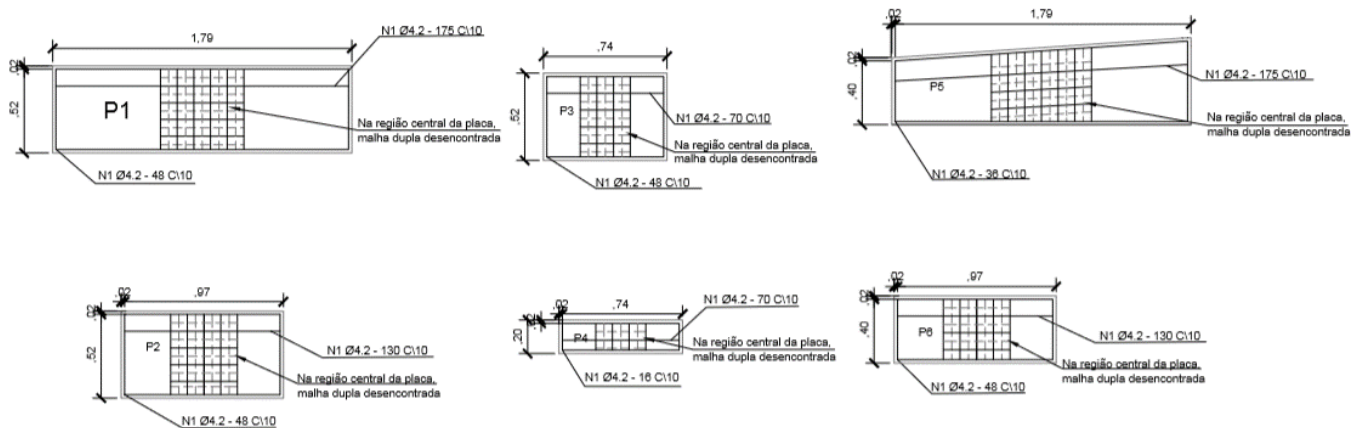
Figura 5: Descrição da malha de ferro
